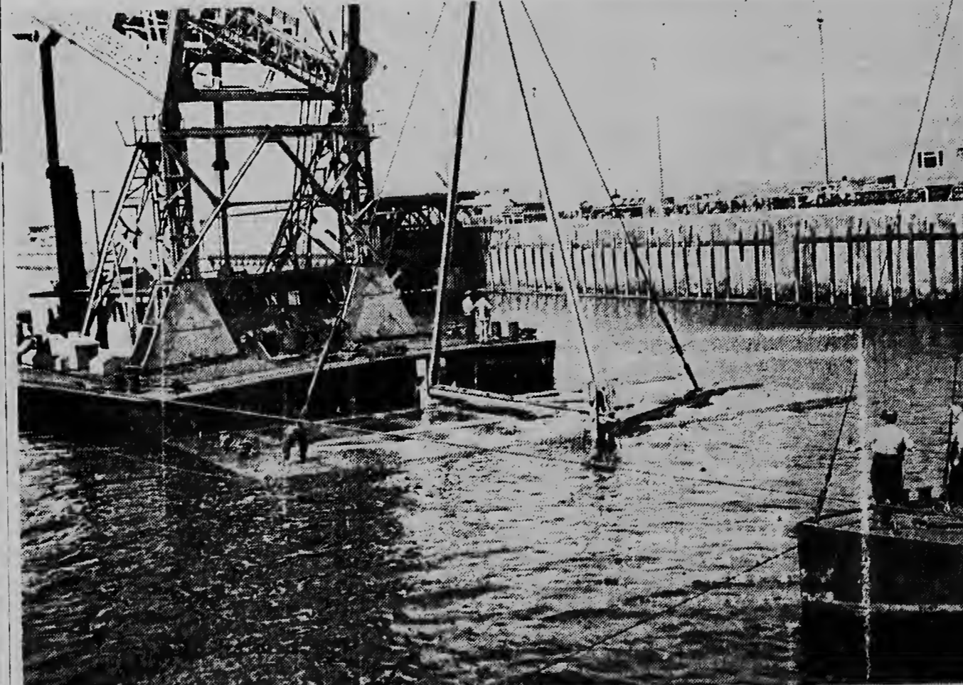
Vanaf 1 september was de Noordersluis in IJmuiden voor alle scheepvaart gesloten in verband met reparatiewerkzaamheden. De foto toont het op zijn plaats brengen van een 110 ton zwaar zinkstuk dat zal moeten dienen als steun voor de zware sluisdeuren.
